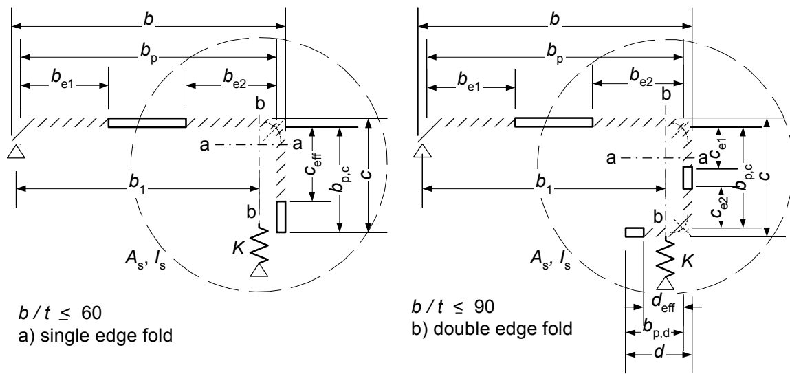
Figure 5.7: Edge stiffeners
